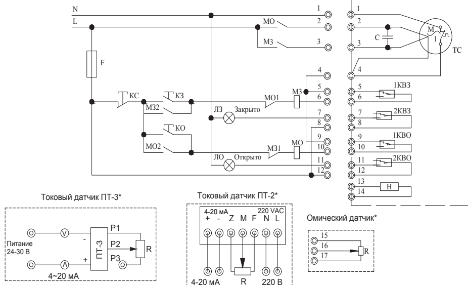
Рис. 2(1). Принципиальная электрическая схема для электроприводов ГЗ-ОФ(К) к сети 220 В, 50 Гц.
