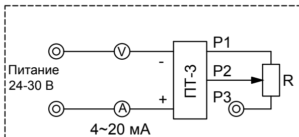
Токовый датчик ПТ-3*
