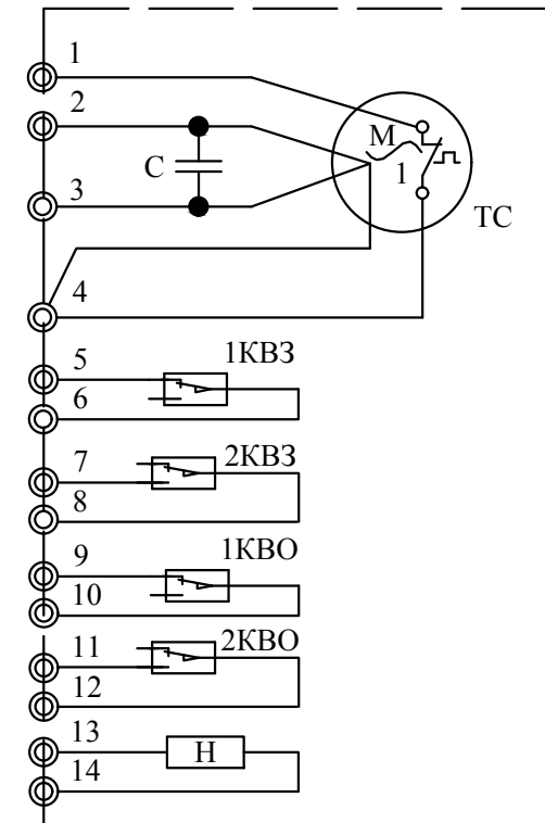
Омический датчик*
