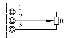
Омический датчик*
