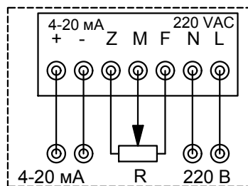
Токовый датчик ПТ-2*
