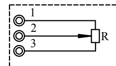
Омический датчик*
