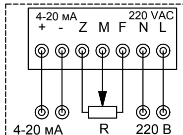
Токовый датчик ПТ-2*
